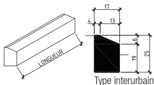
Type interurbain
