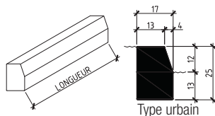
Type urbain
